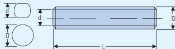
Durostone®-螺杆
