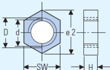
Durostone®-六角螺母
