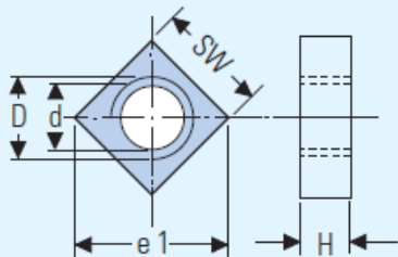
Durostone®-方螺母
